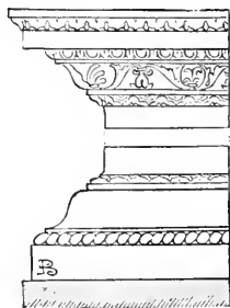
Fig. 636. Stylobates.
